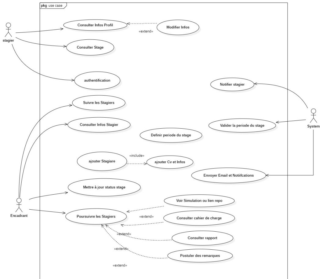
FIGURE 7.1 – Figure 4.2 : : Diagramme de cas d'utilisation : trois rôles et interactions
